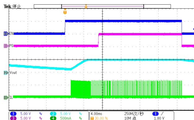
Figure 16. Enable (Iload=10mA)
