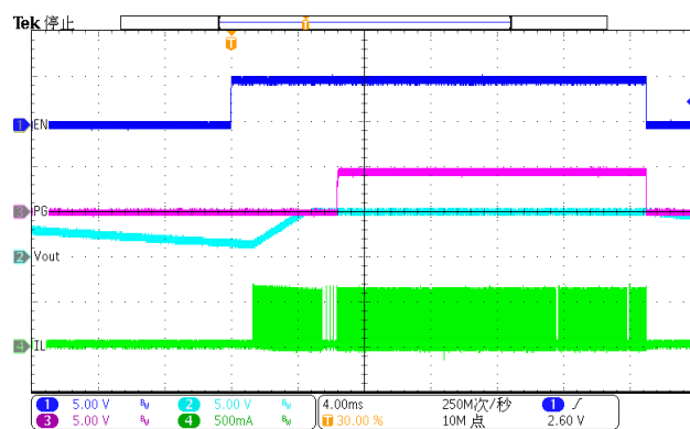
Figure 16. Enable (Iload=10mA)
