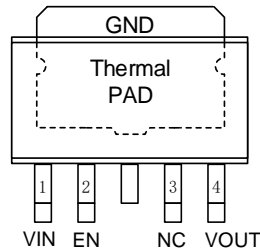
SCT71405FxxQOWCR
